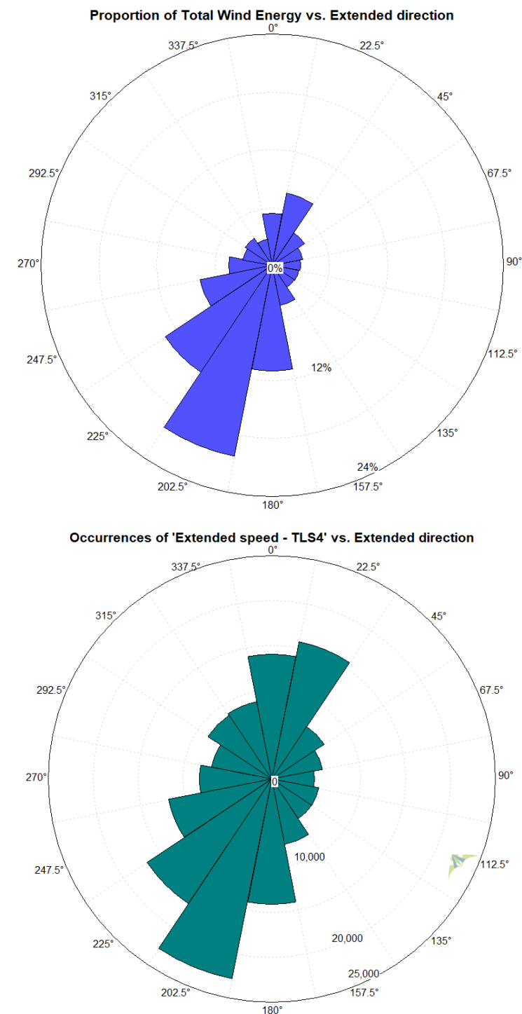
Figure 3 : Rose des vents. Fréquence des vents en vert, puissance des vents en bleu (Source : ELEMENTS, 2019)
